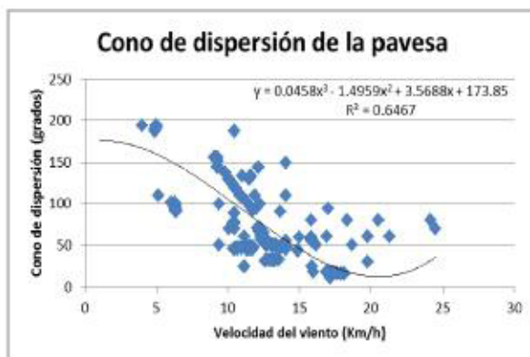
Figura 5. Cono de dispersión y desplazamiento de la pavesa cuando el viento tiene velocidad de 18 km/h y 10 km/h. Fuente: ICC, 2014.
