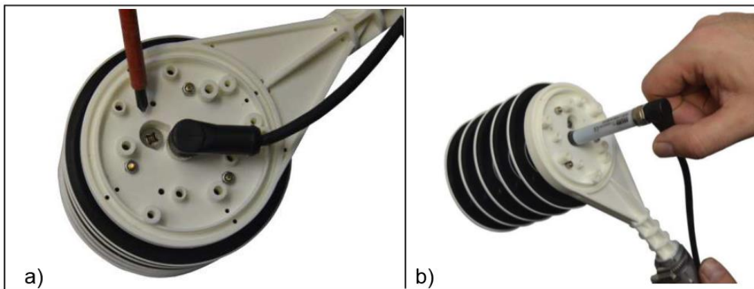
Figura 71. a) Ubicación de tornillo, b) Proceso para retirar el sensor TR1
