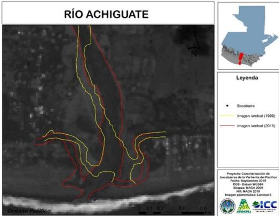
Fuente elaboración propia, 2015. Figura 96A. Bocabarra río Achiguate
