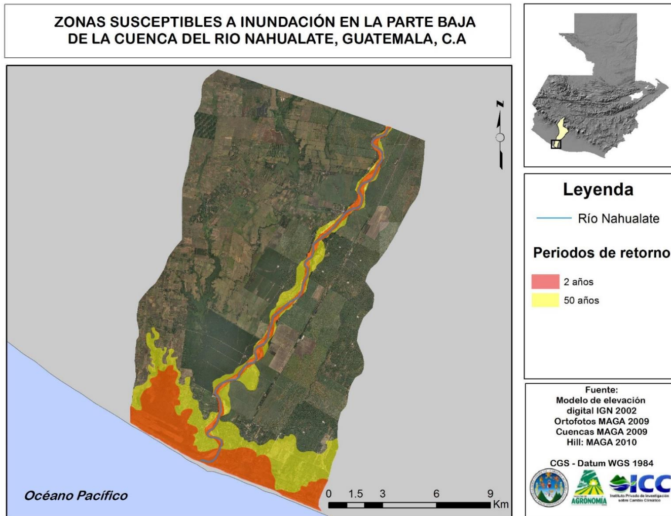
Figura 40. Zonas susceptibles a inundaciones en la parte baja de la cuenca del río Nahualate
