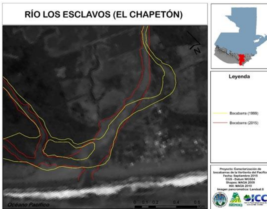
Fuente elaboración propia, 2015. Figura 101A. Bocabarra río Los Esclavos (El Chapetón)
