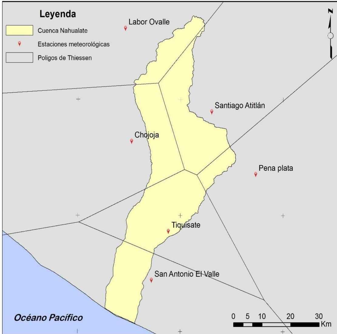
Figura 16. Área de influencia de las estaciones Labor Ovalle. Chojaja. Santiago Atitlán. Peña Plata. Tiquisate. San Antonio El Valle, a partir de polígonos de Thiessen
