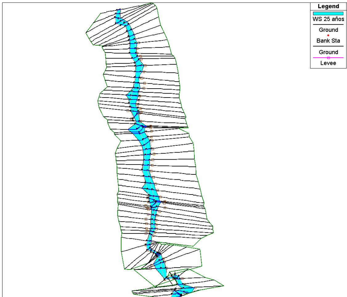
Fuente: elaboración propia, 2015. Figura 34. Vista de planta de simulación hidráulica del río Nahualate en la zona de estudio (T: 25 años).
