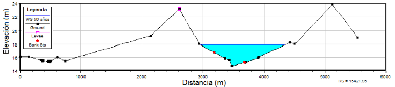
Figura 37. Perfil de una sección del río (T: 50 años)
