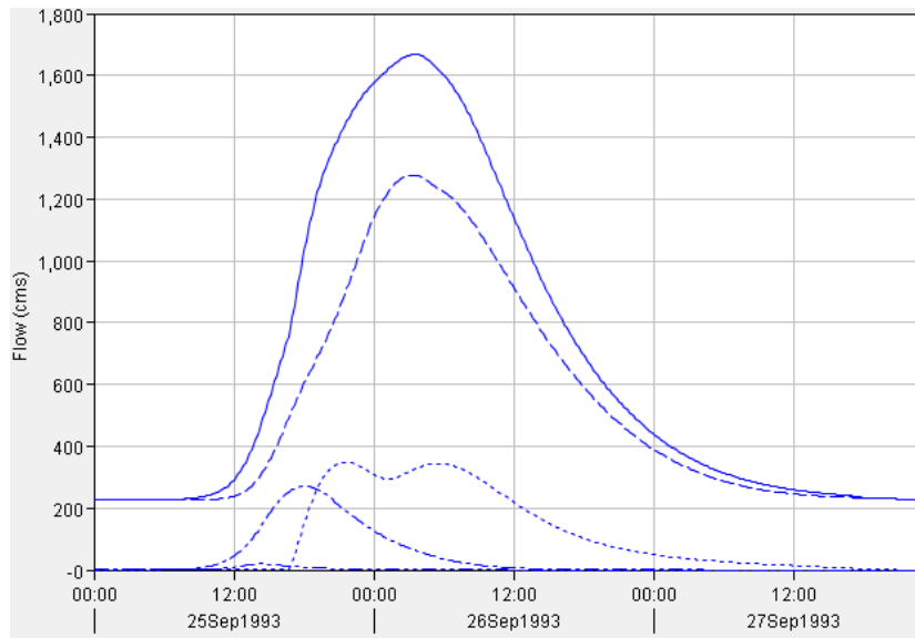
Figura 47A. Hidrograma generado en el modelo hidrológico para el punto de entrada de la zona de estudio, correspondiente a un periodo de retorno de 5 años.
