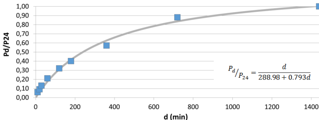
Figura 14. Gráfica de los valores observados y calculados mediante la ecuación adoptada para el periodo de retorno de 136 años.
