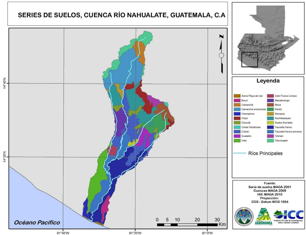
Figura 17. Series de suelo presentes en la cuenca del río Nahualate
