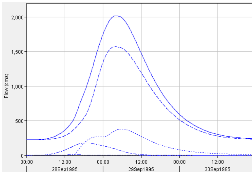
Figura 46A. Hidrograma generado en el modelo hidrológico para el punto de entrada de la zona de estudio, correspondiente a un periodo de retorno de 2 años.
