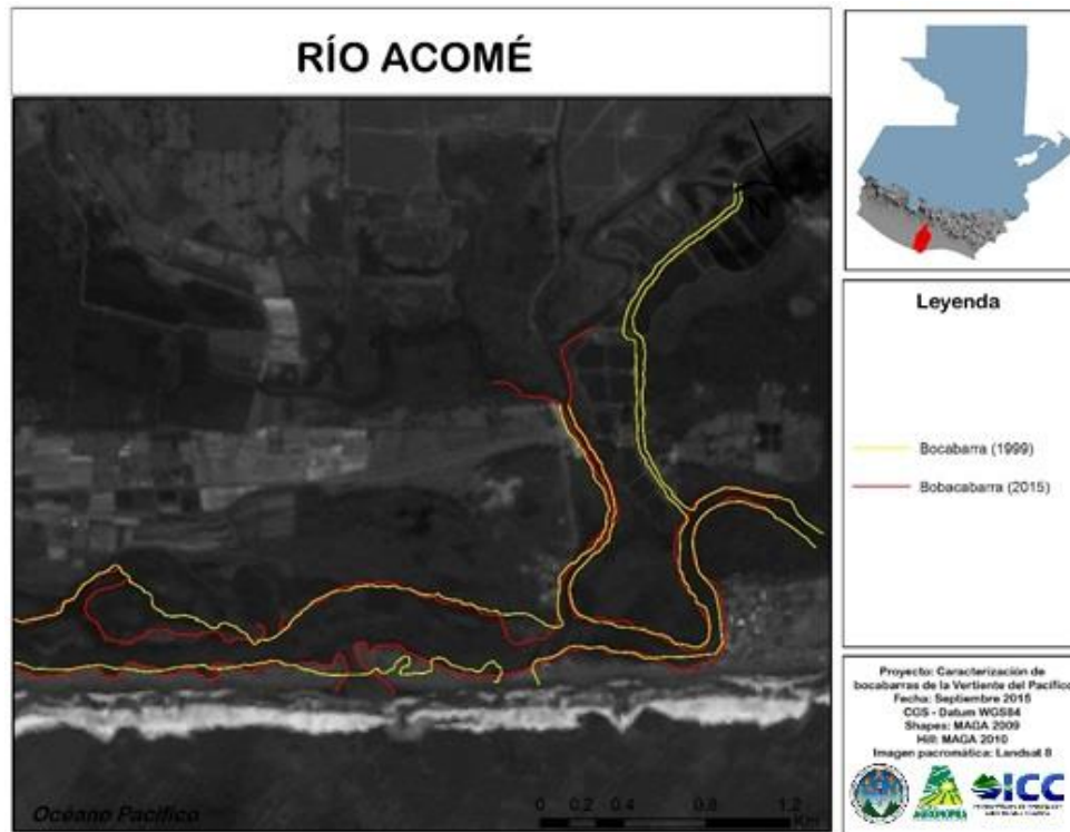
Fuente elaboración propia, 2015. Figura 95A. Bocabarra río Acomé
