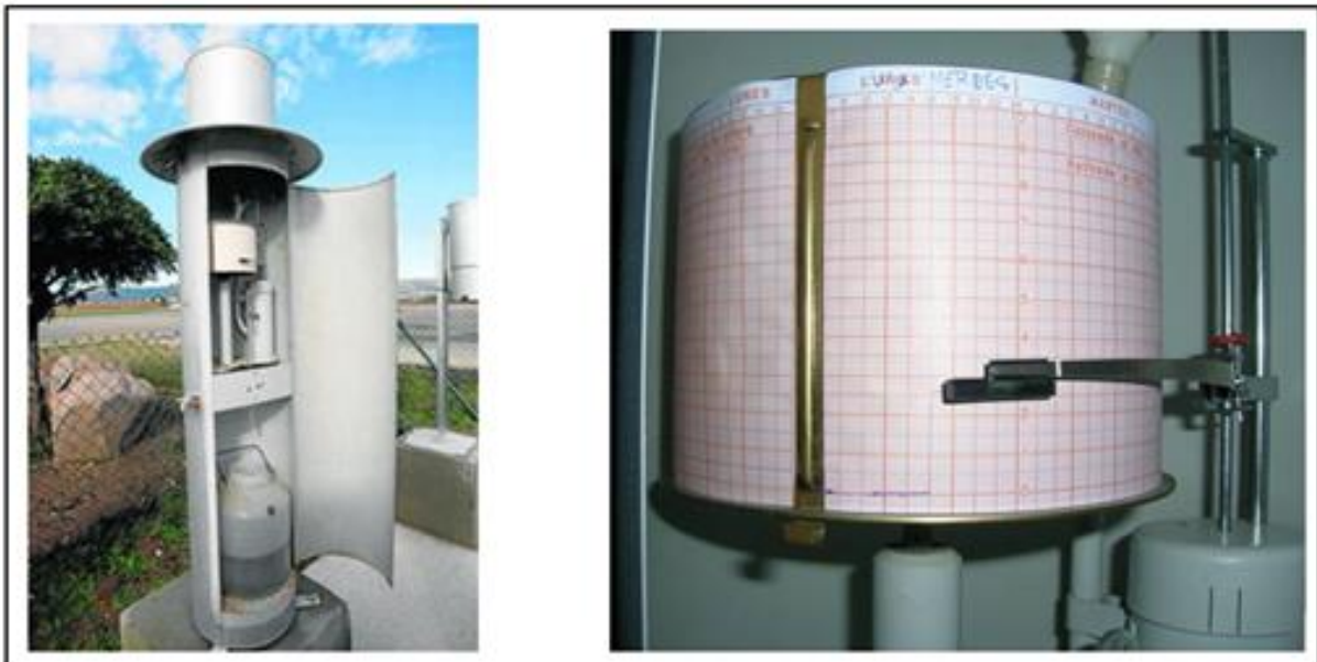
Figura 8. Imagen correspondiente a un pluviógrafo. Nótese como la pluma registra el incremento de la precipitación a lo largo del tiempo (intensidad de lluvia).
