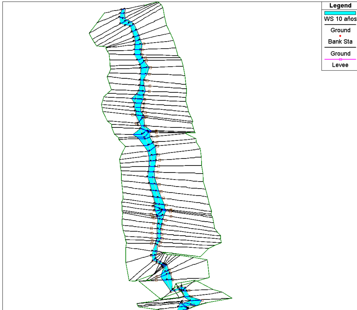
Fuente: elaboración propia, 2015. Figura 32. Vista de planta de simulación hidráulica del río Nahualate en la zona de estudio (T: 10 años).
