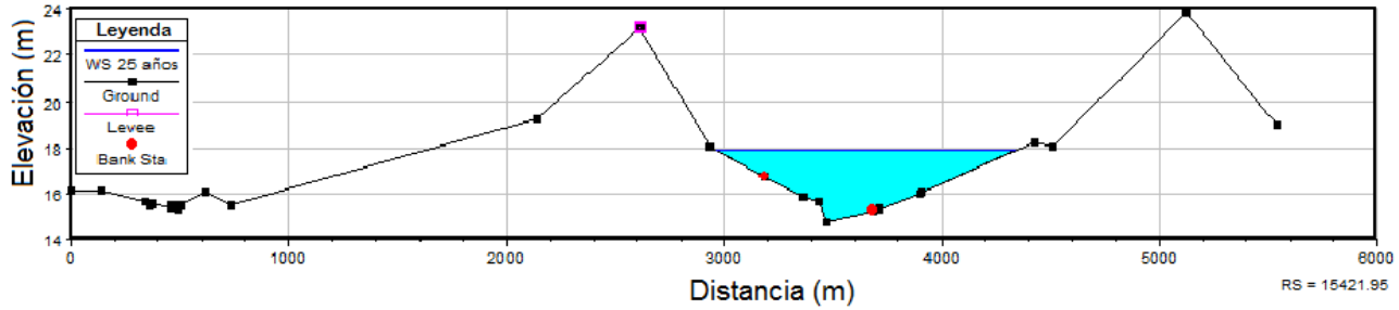
Figura 35. Perfil de una sección del río (T: 25 años)
