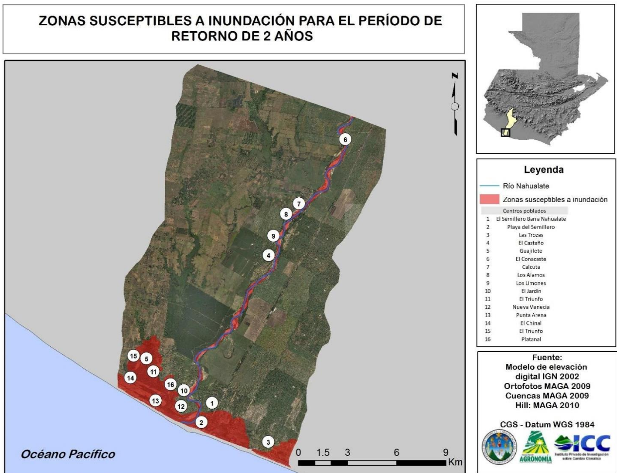
Figura 38. Centros poblados y superficie inundable para el periodo de retorno de 2 años.
