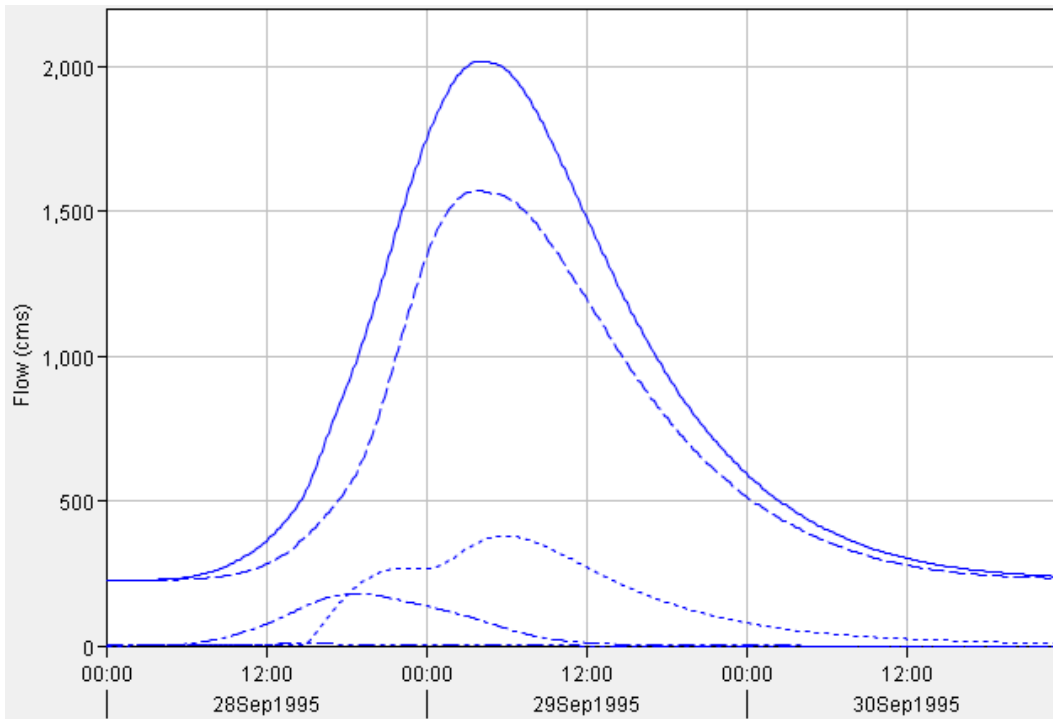
Figura 27. Hidrograma generado en el modelo hidrológico para el punto de entrada de la zona de estudio, correspondiente a un periodo de retorno de 50 años.
