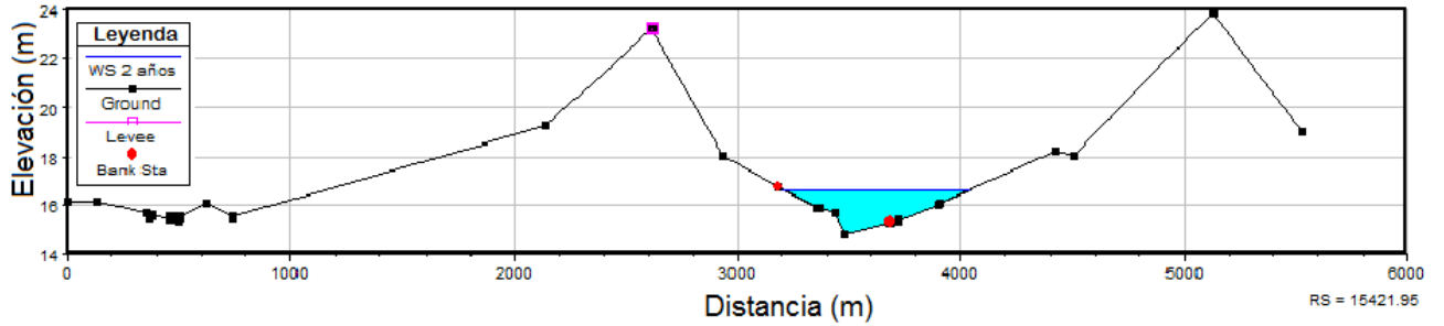
Fuente: elaboración propia, 2015. Figura 29. Perfil de una sección del río (T: 2 años)
