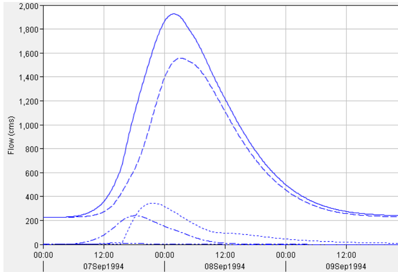
Figura 49A. Hidrograma generado en el modelo hidrológico para el punto de entrada de la zona de estudio, correspondiente a un periodo de retorno de 25 años.
