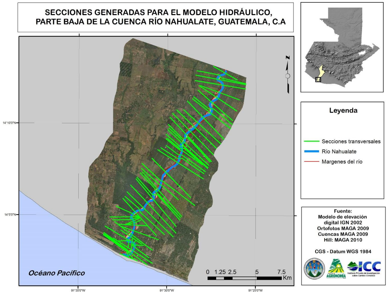
Figura 21. Secciones generadas a partir del modelo de elevaciones del terreno.
