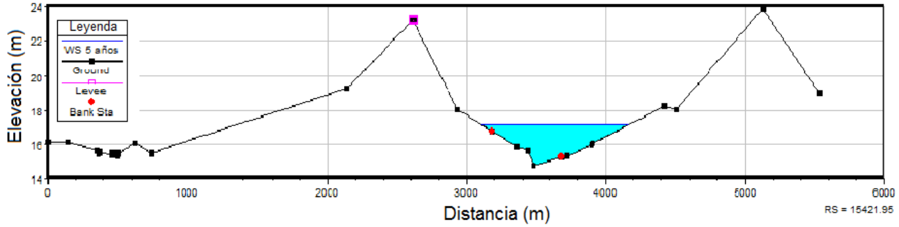
Fuente: elaboración propia, 2015. Figura 31. Perfil de una sección del río (T: 5 años)
