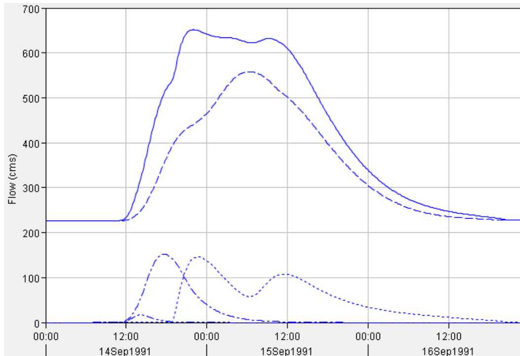
Figura 26. Hidrograma generado en el modelo hidrológico para el punto de entrada de la zona de estudio, correspondiente a un periodo de retorno de 2 años. Nótese que este hidrograma es la suma de todos los hidrogramas procedentes de las subcuencas.
