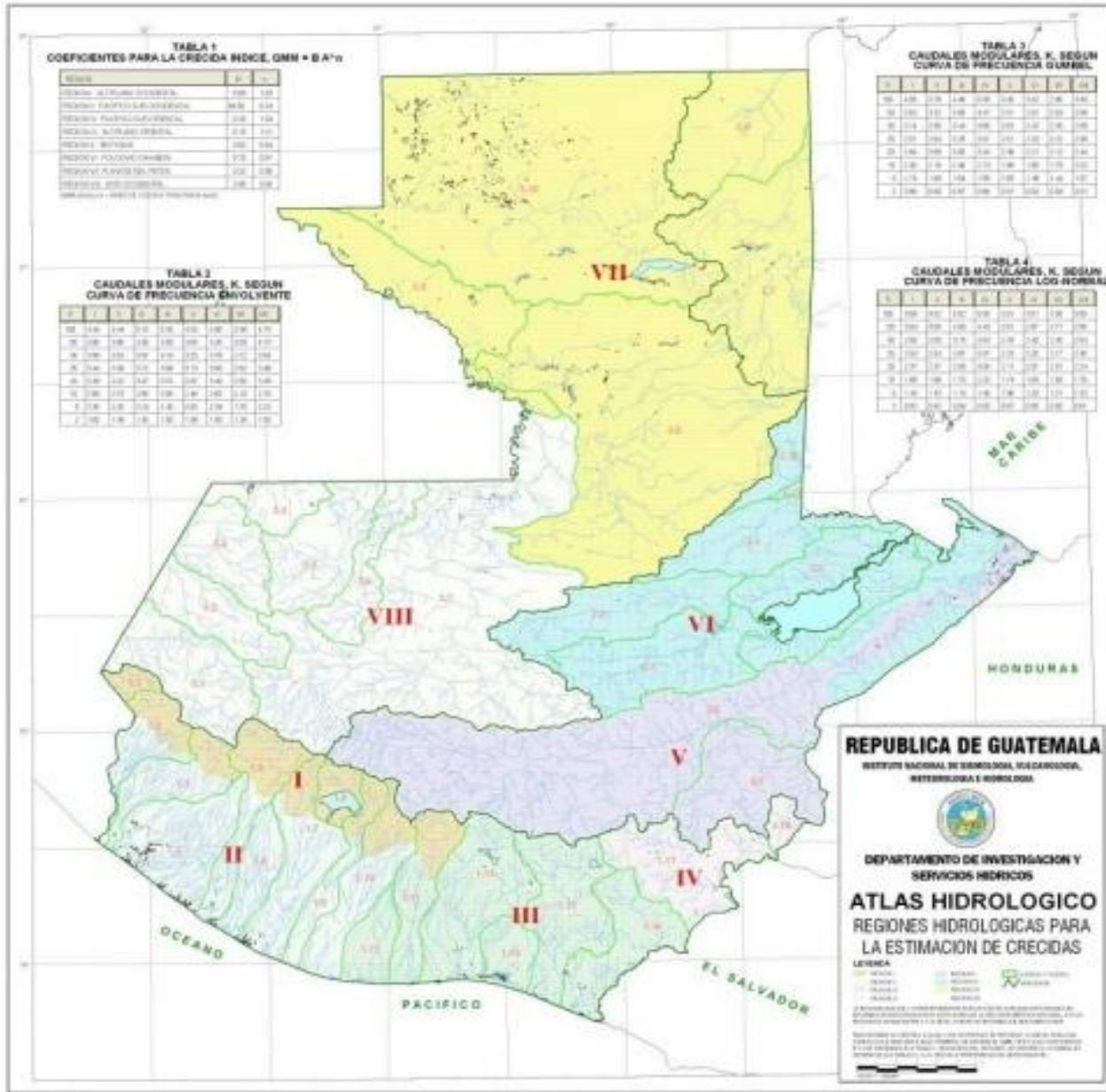
Figura 20. Regiones hidrológicas para la estimación de crecidas en Guatemala
