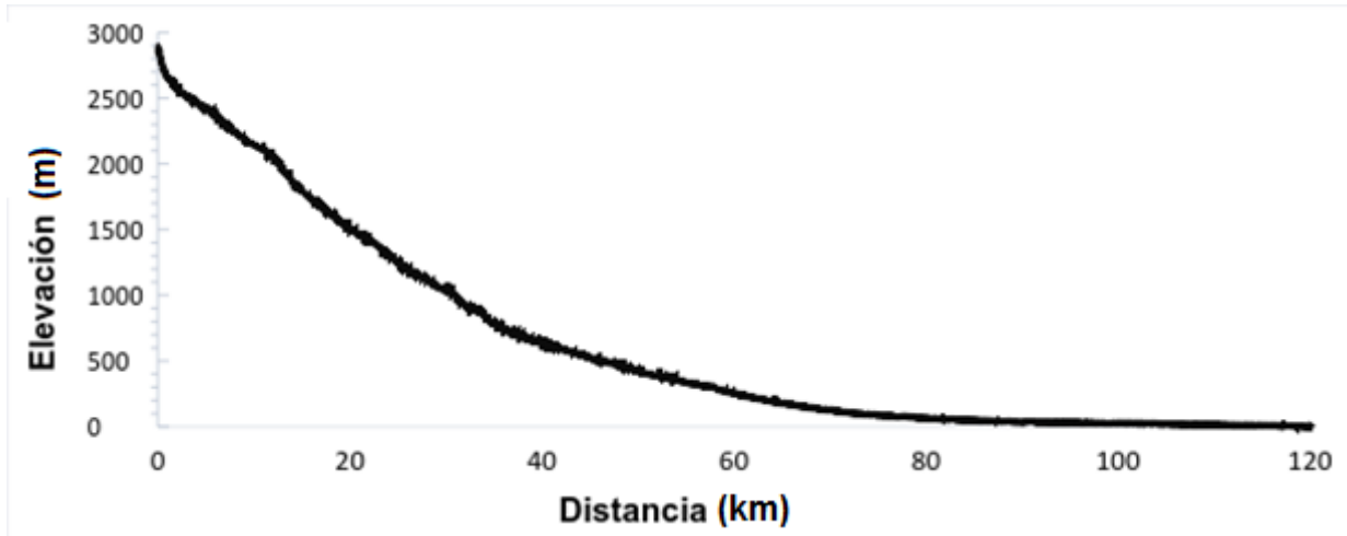
Figura 10. Perfil longitudinal del cauce del río Nahualate
