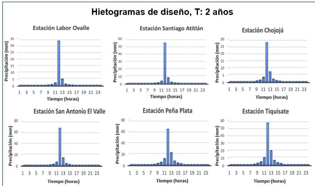
Figura 41A. Hietogramas de diseño para cada una de las estaciones para el periodo de retorno de 2 años generados a partir de las ecuaciones generadas por el método de Mendoza.
