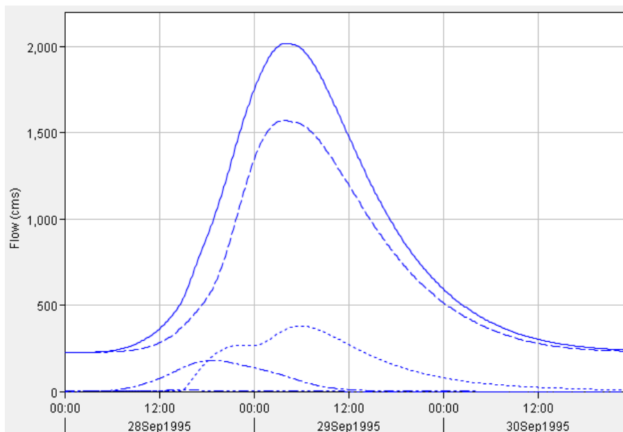
Figura 50A. Hidrograma generado en el modelo hidrológico para el punto de entrada de la zona de estudio, correspondiente a un periodo de retorno de 50 años
