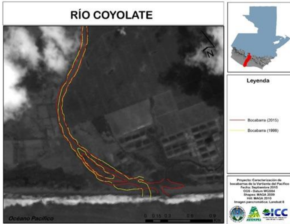
Fuente elaboración propia, 2015. Figura 94A. Bocabarra río Coyolate
