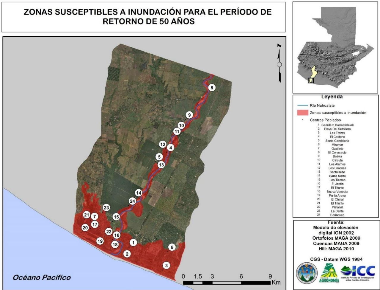
Figura 39. Centros poblados y superficie inundable para el periodo de retorno de 50 años
