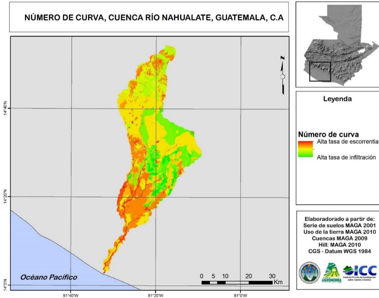
Figura 18. Distribución del parámetro de número de curva, en la cuenca del río Nahualate.
