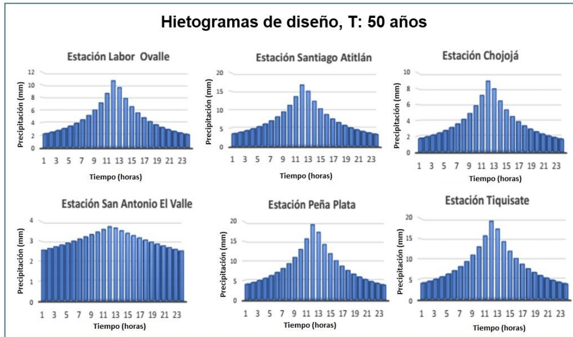
Figura 45A. Hietogramas de diseño para cada una de las estaciones para el periodo de retorno de años generados a partir de las ecuaciones generadas por el método de Mendoza.
