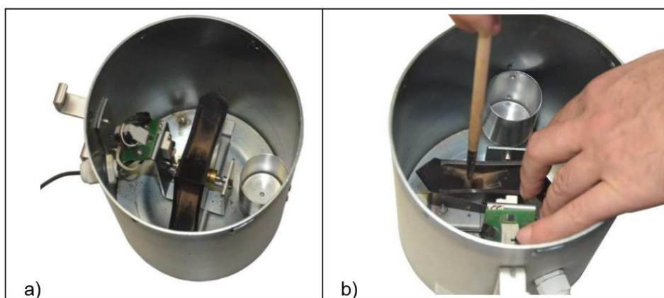
Figura 68. a) Interior de pluviómetro con residuos de arena, b) Limpieza del interior del pluviómetro
