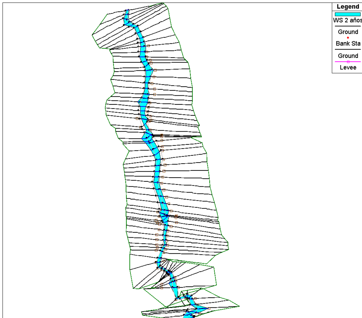
Figura 28. Vista de planta de simulación hidráulica del río Nahualate dentro de la zona de estudio (T: 2 años).
