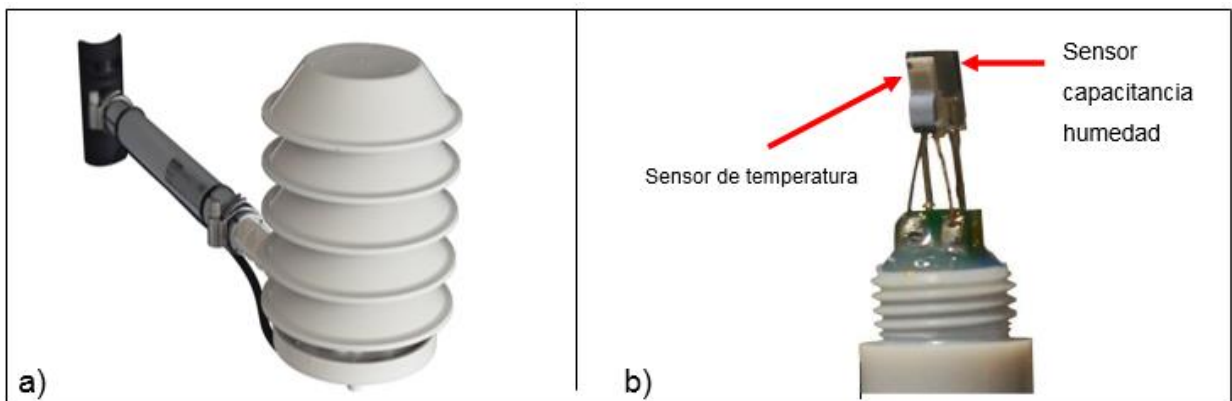
Figura 61. a) Escudo protector, b) sensores de temperatura y humedad
