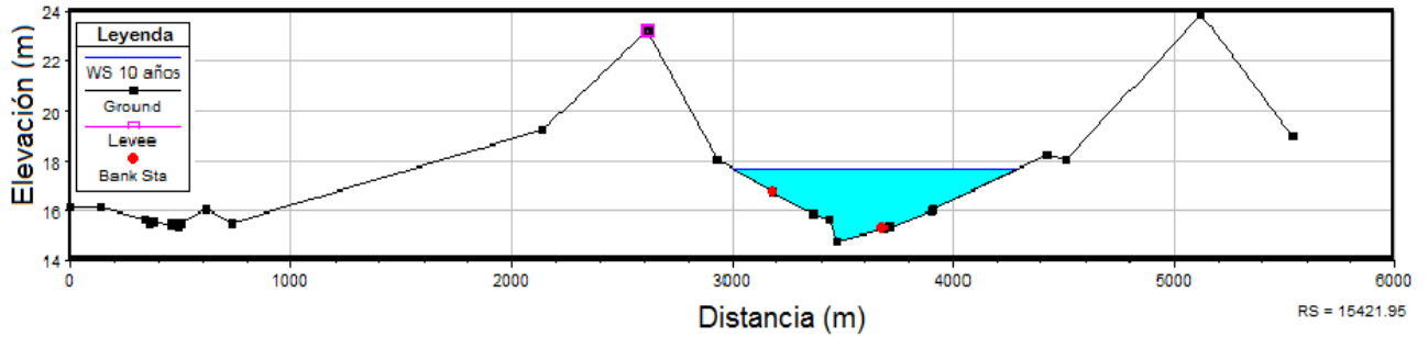
Fuente: elaboración propia, 2015. Figura 33. Perfil de una sección del río (T: 10 años)
