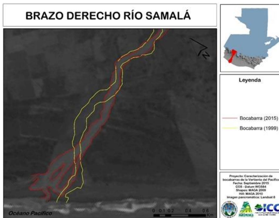
Fuente: elaboración propia, 2015. Figura 85A. Bocabarra brazo derecho río Samalá
