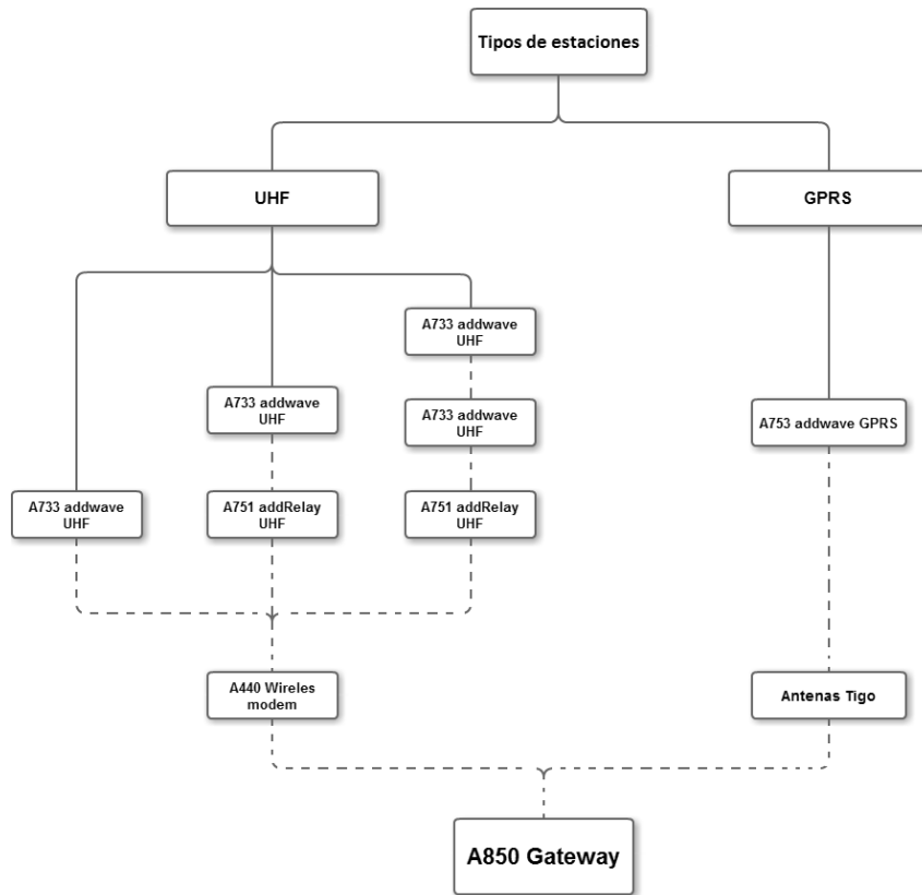
Figura 51. Diagrama de transmisión de datos en las estaciones UHF y GSM/GPRS Ubicación de las estaciones de la red meteorologica del ICC.
