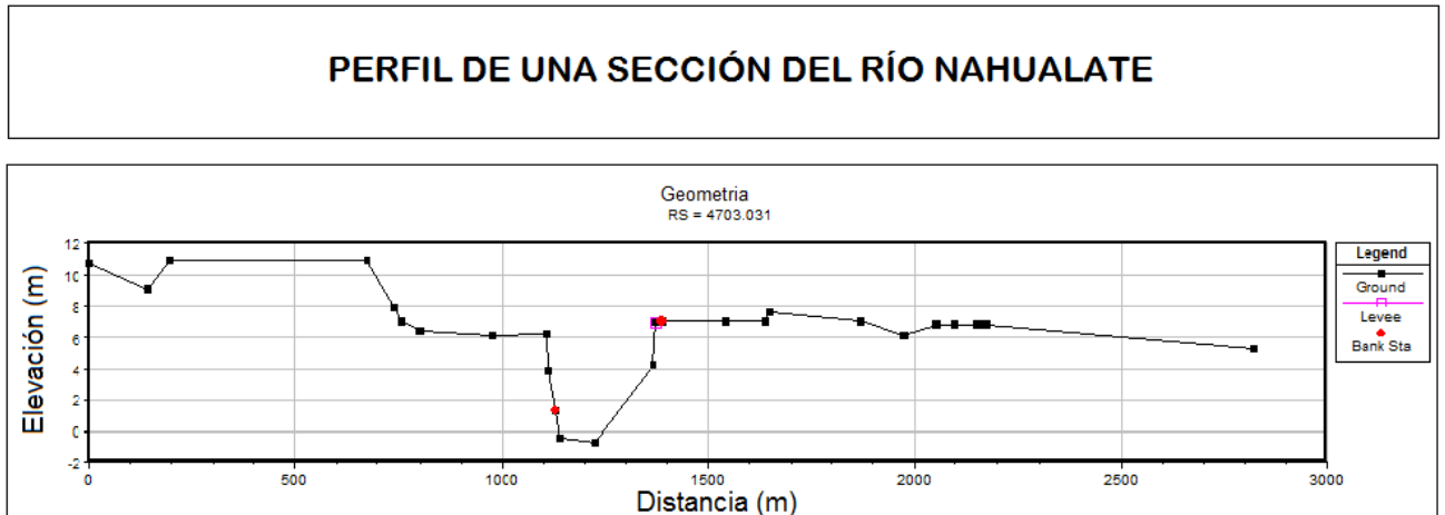
Figura 23. Vista de perfil de una sección de la geometría del río Nahualate.
