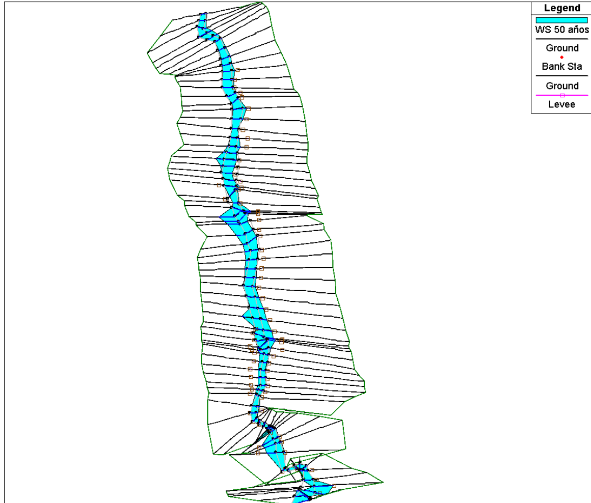
Figura 36. Vista de planta de simulación hidráulica del río Nahuatlato en la zona de estudio (T: 50 años).
