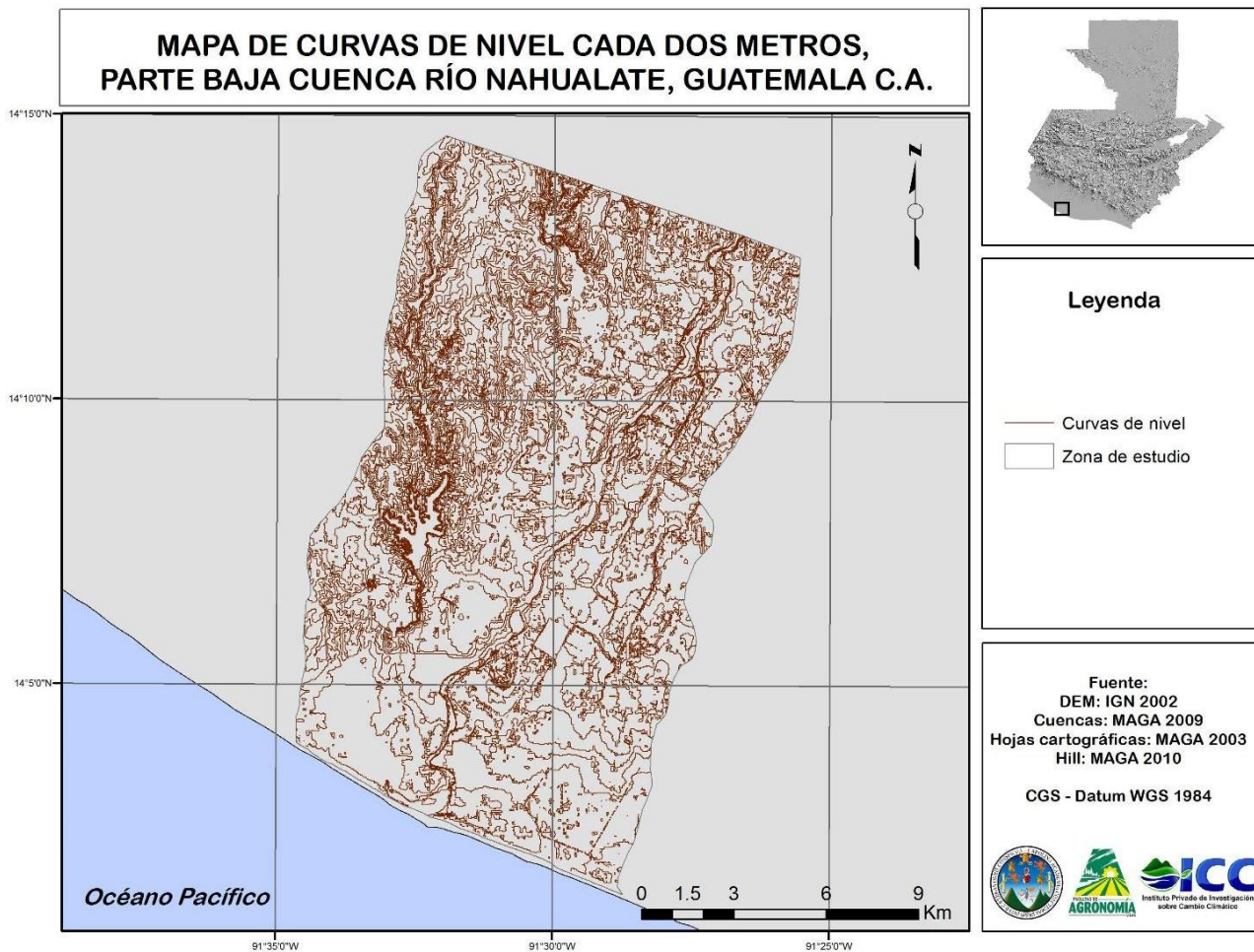
Figura 24. Topografía del terreno obtenida a partir del MED, para la delimitación de zonas inundables
