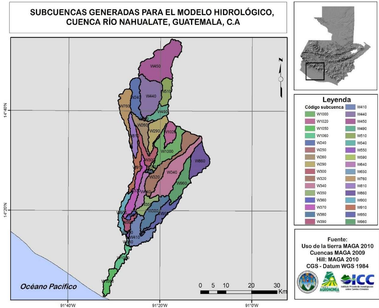
Figura 19. División de la cuenca Nahualate en subcuencas para la generación del modelo hidrológico.
