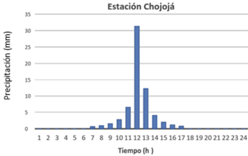
Figura 25. Hietograma de diseño para un periodo de 5 años para la estación de Chojója.
