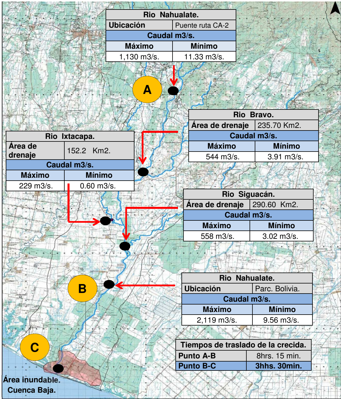
Mapa 22. Puntos propuestos para implementar un sistema de monitoreo de crecidas.
