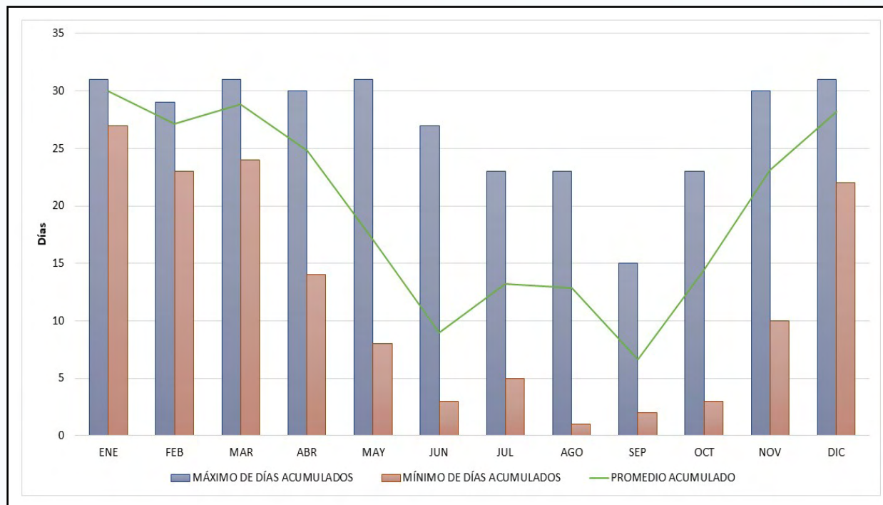
Figura 14. Comportamiento de los días acumulados sin lluvia en el municipio de San José Chacayá. Fuente: (INSIVUMEH, 2021).
