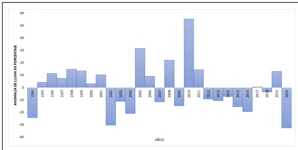
Figura 7. Anomalía de la precipitación en función al promedio acumulado mensual para el período 1994-2020, estación meteorológica de Santa María El Tablón.
