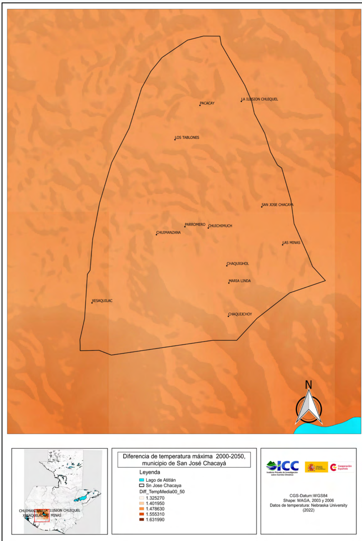
Figura 21. Diferencia de temperatura máxima para el periodo 2000-2050 en el municipio de San José Chacaya. Fuente: University of Nebraska-Lincoln, (2022)
