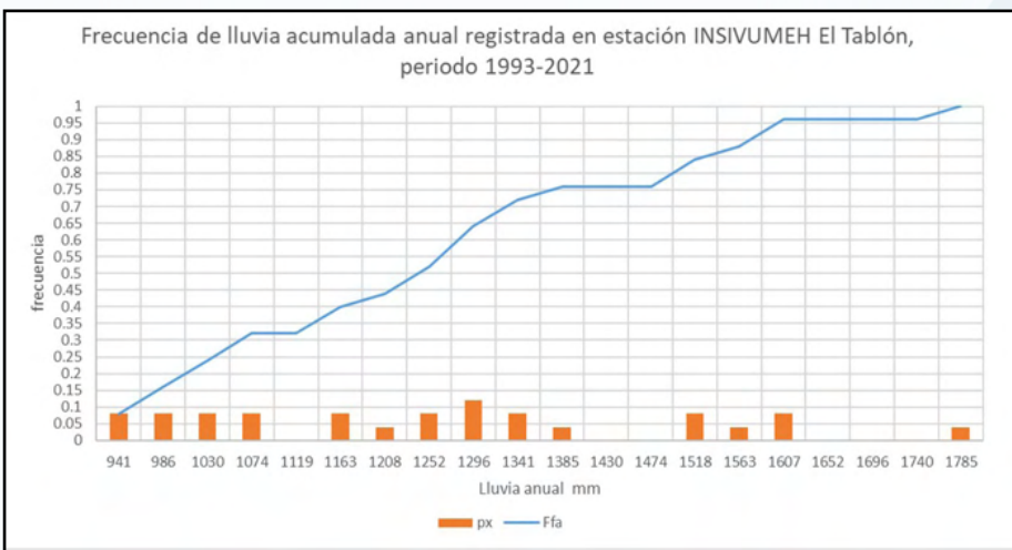
Figura 9. Frecuencia de ocurrencia de lluvia acumulada anual registrada en la estación Santa María El Tablón. Fuente: INSIVUMEH (2021)
