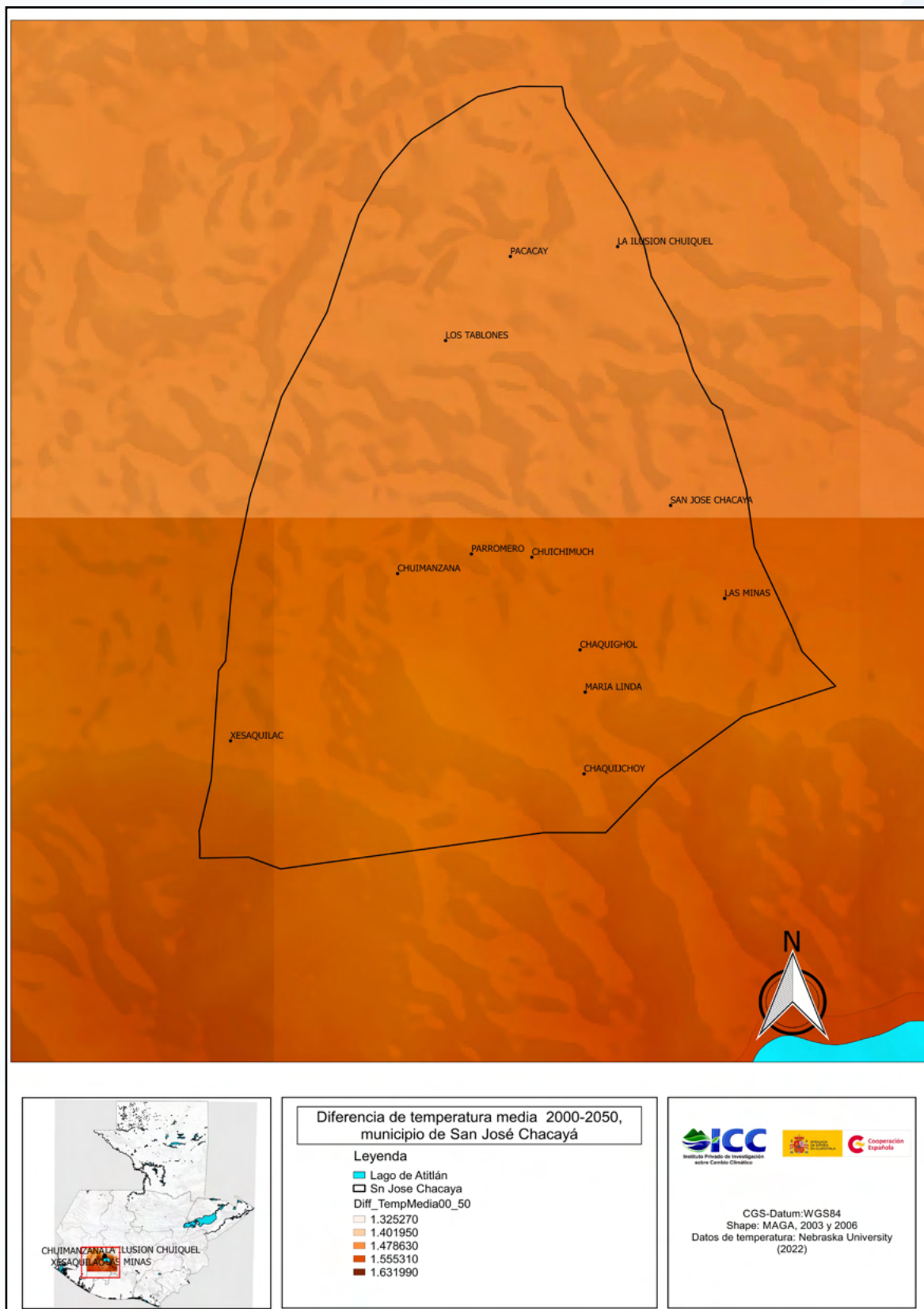
Figura 22. Diferencia de temperatura media para el período 2000-2050 en el municipio de San José Chacayá. Fuente: (University of Nebraska-Lincoln, 2022).
