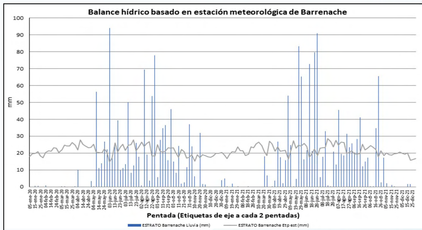
Figura 10. Balance hídrico para el municipio de San José Chacayá basado en datos de la estación meteorológica de Barreneché. Fuente: AMSCLAE (2022).
