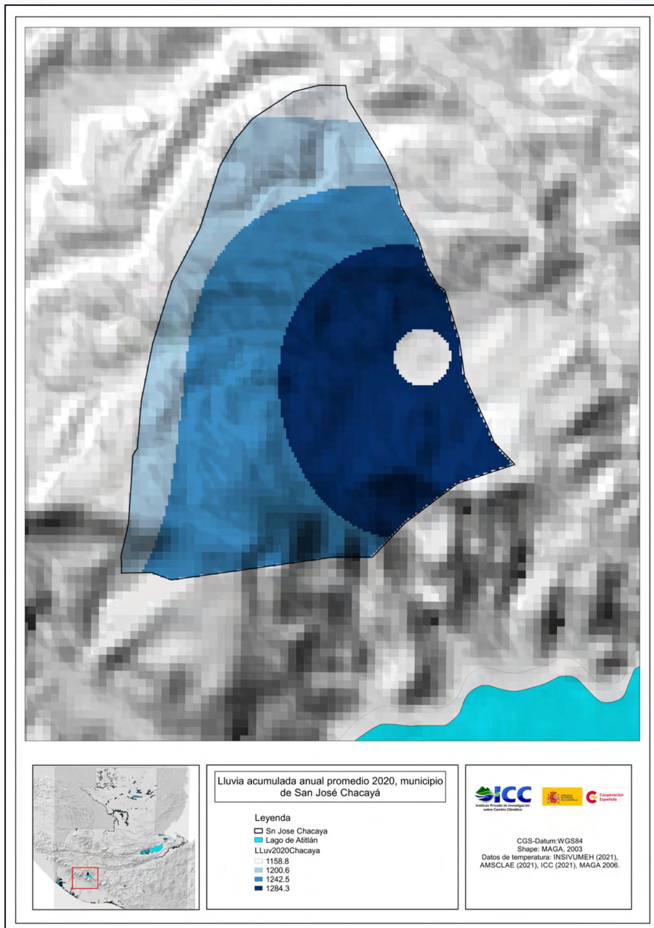
Figura 5. Distribución espacial de precipitación (lluvia) acumulada 2020 en el municipio de San José Chacayá. Fuente: INSIVUMEH (2021), AMSCLAE (2021), ICC (2021).
