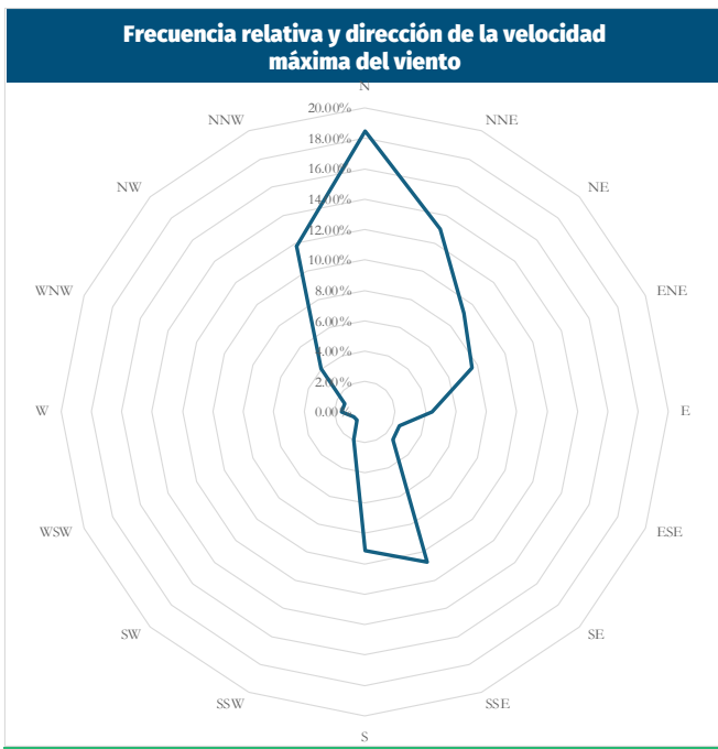
Figura 17. Dirección de los vientos con máxima velocidad registrada para el territorio de El Rosario, Sololá. Fuente: Elaborado con datos de estación meteorológica El Tablón AMSCLAE.
